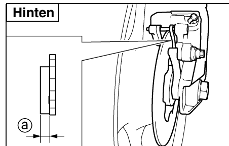
a. Bremsbelag-Stärke
