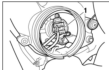
1. Scheinwerfer-Steckverbinder
