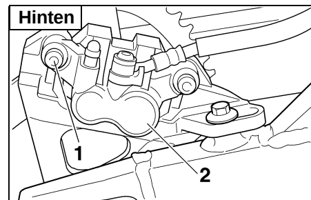
1. Schraube 2. Bremssattel
