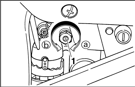
1. Einstellschraube (Druckstufen-Dämpfungskraft)
