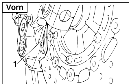
1. Scheibenbremsbelag-Verschleißanzeiger
